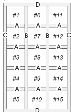
Plano de material para tiras
