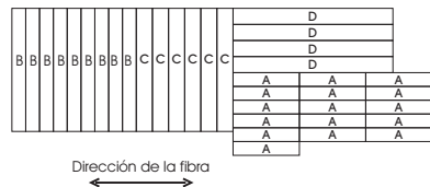
Plano de material para tiras
