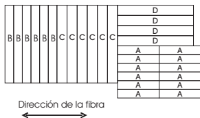
Plano de material para tiras
